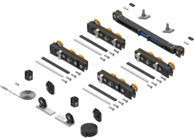
SV-Sincro Q110 Fitting set. x1 Double SofTop
